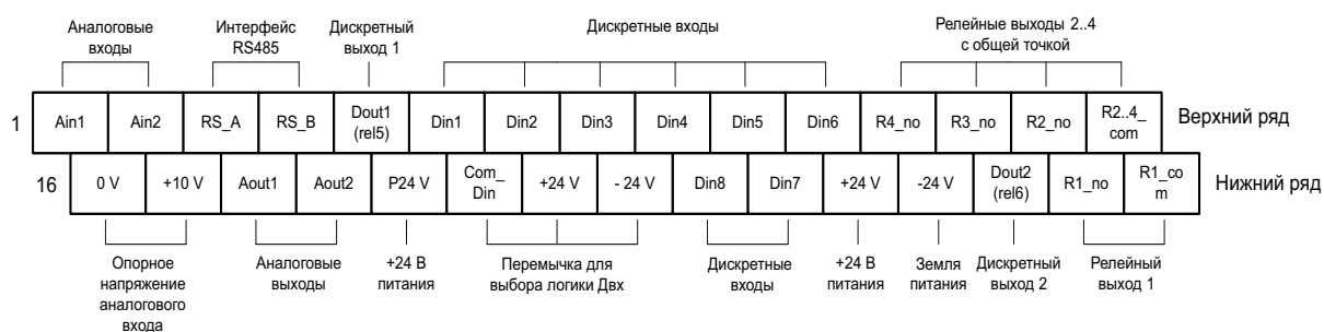
Рисунок 2.10 — Назначение контактов разъёма подключения периферии
