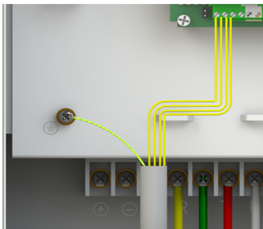
Рисунок 2.11 — Заземление кабеля управления, типоразмер (11К-18К)
