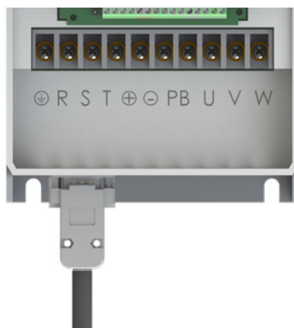
Рисунок 2.12 — Подключение кабеля энкодера , типоразмер (5К5-7К5)
