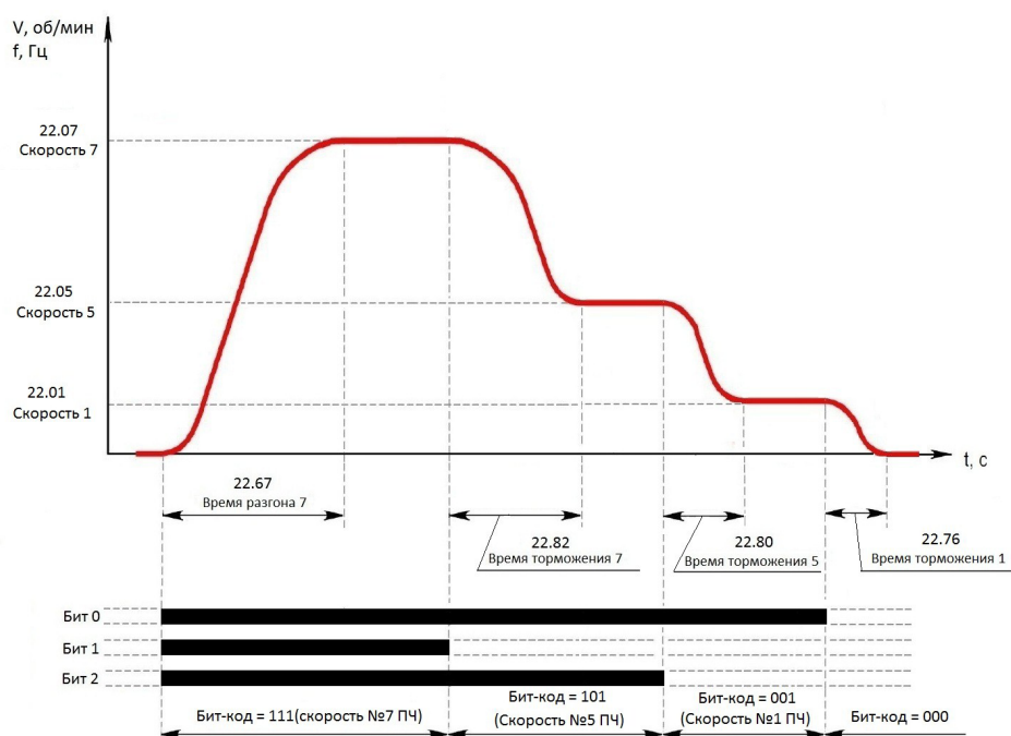
Рисунок 4.2 – Пример профиля S-образной характеристики разгона и торможения штатного движения кабины лифта при трехскоростной станции управления.
