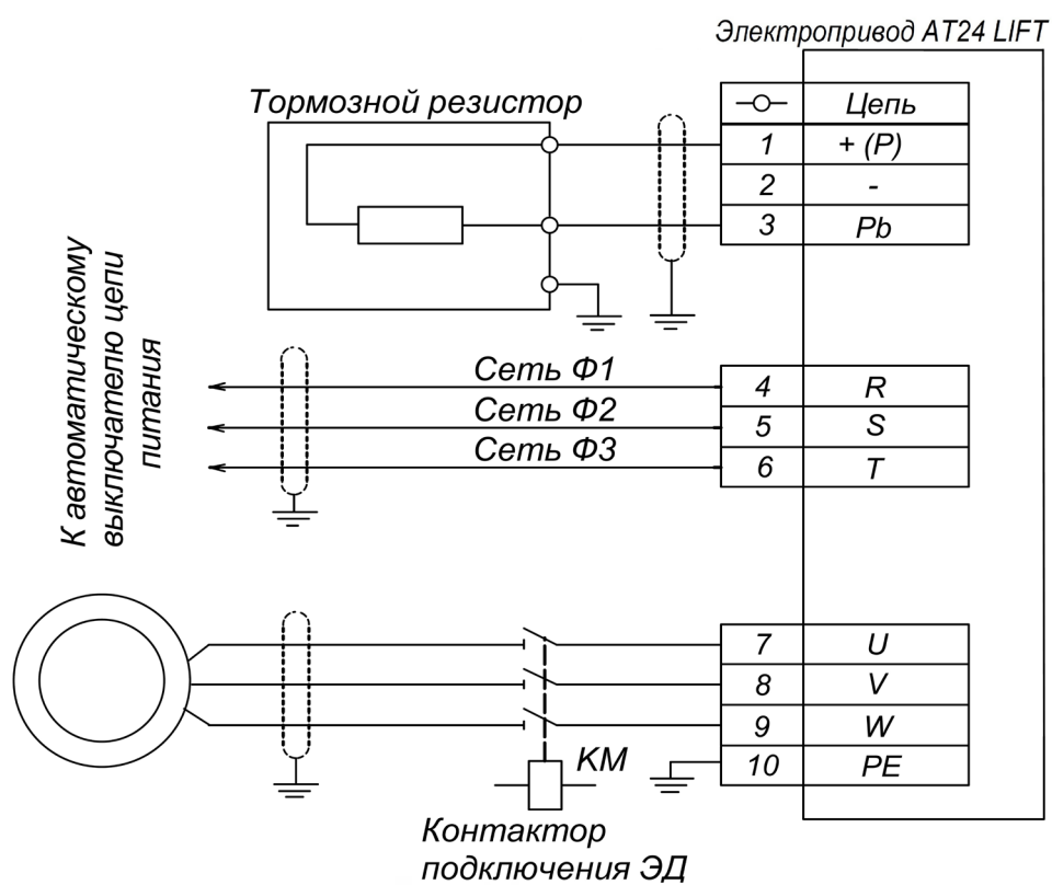
Рисунок 2.18 — Подключение силовых цепей к электроприводу Триол AT24 ЛИФТ 11к...18к
