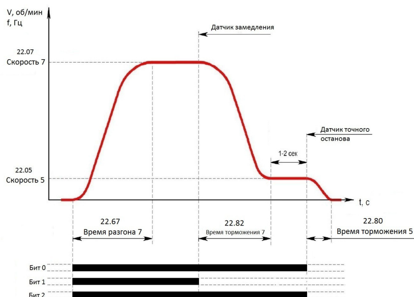
Рисунок 4.1 – Пример профиля S-образной характеристики разгона и торможения штатного движения кабины лифта при двухскоростной станции управления
