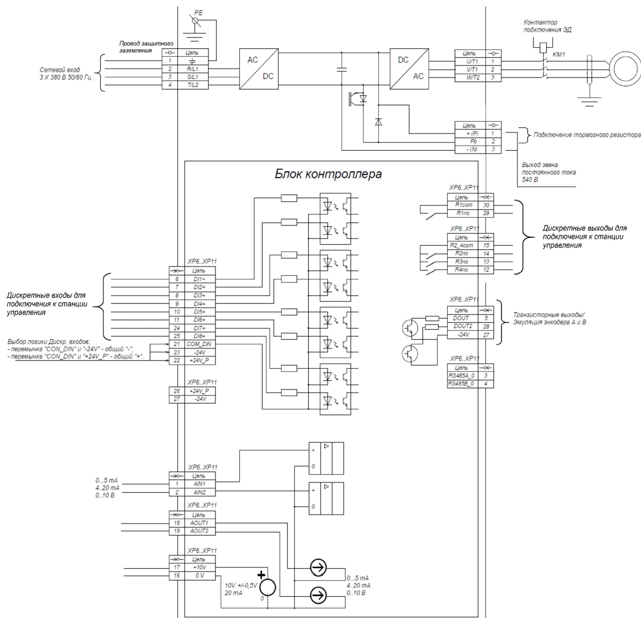
Рисунок 2.16 — Общая схема внешних подключений к электроприводу Триол AT24 ЛИФТ
