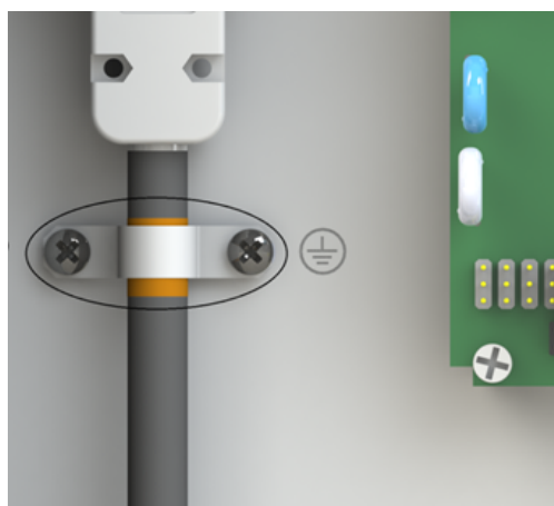
Рисунок 2.13 — Подключение и заземление кабеля энкодера , типоразмер (11К-18К)
