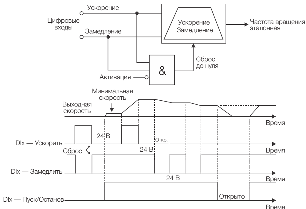
Рисунок 19.28. Работа функции электронного потенциометра (EP)
