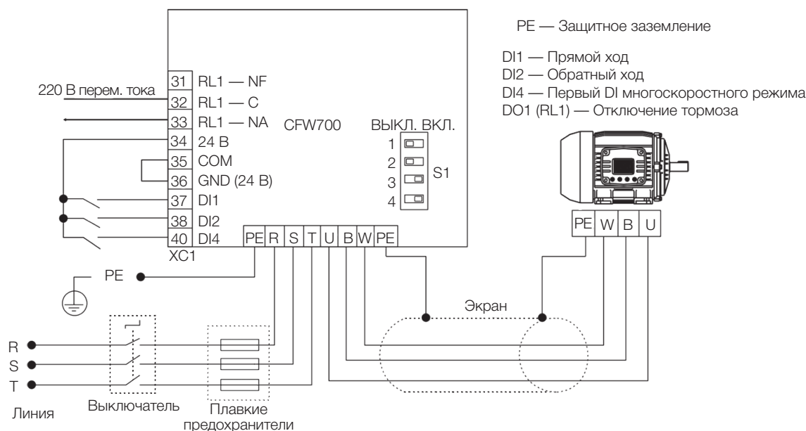
Рисунок 19.38. Пример работы функции логической последовательности работы механического тормоза в преобразователе CF700
