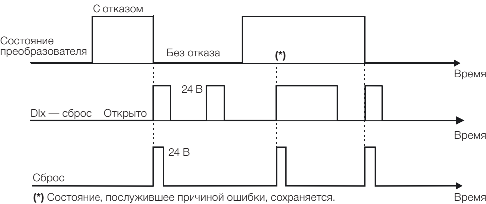
Рисунок 13.5.(а) – (j) Подробное описание работы функций цифровых входов
