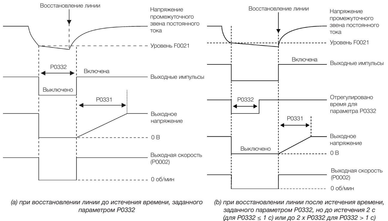
Рисунок 12.5.(a) и (b) Функция компенсации провалов напряжения в сети в режиме V/f или VVW
