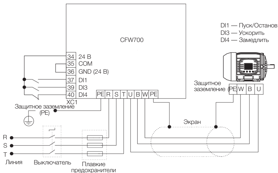
Рисунок 19.7. Пример работы приложения электронного потенциометра в CFW700
