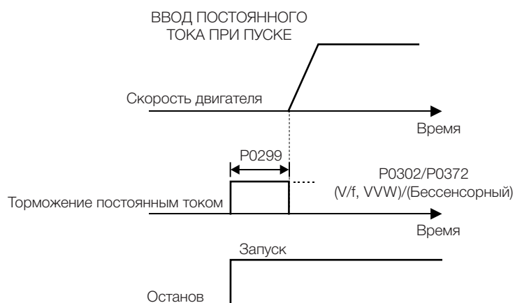
Рисунок 12.8. Использование торможения постоянным током при пуске
