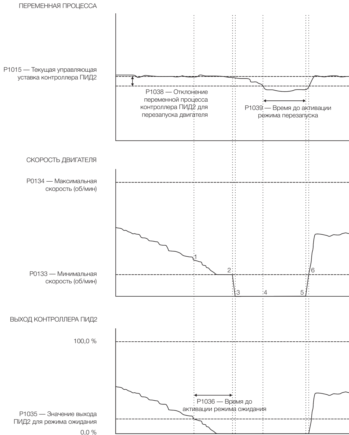
Рисунок 19.24. Работа ПИД2 в режиме ожидания и режиме перезапуска
