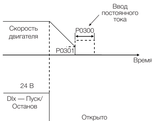
Рисунок 12.9. (a) и (b) Использование торможения постоянным током при отключении кривой (посредством отключения кривой)
