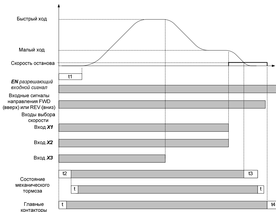
Рисунок 22. Временная диаграмма сигнала для нормального перемещения.
