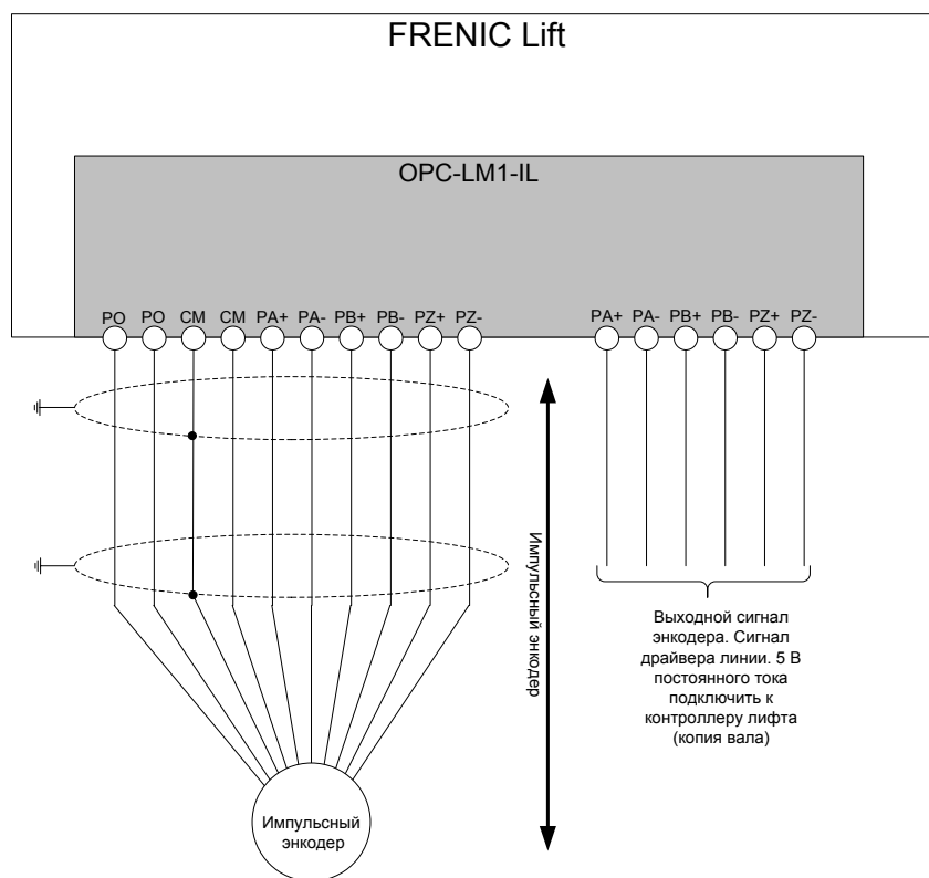
Рисунок 9. Соединение с дополнительной платой.
