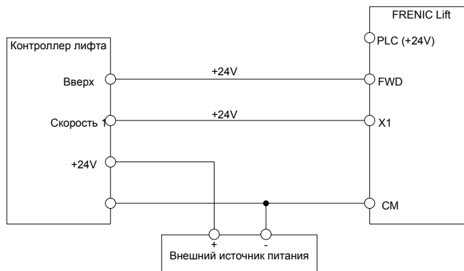
Рисунок 4. Соединение с использованием внешнего источника питания.
